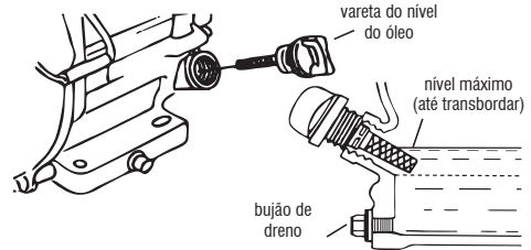
Fig. 7 – Nível de óleo
