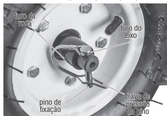
Fig. 6 – Instalação das rodas
