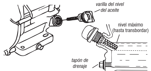
Fig. 7 – Nivel de aceite
