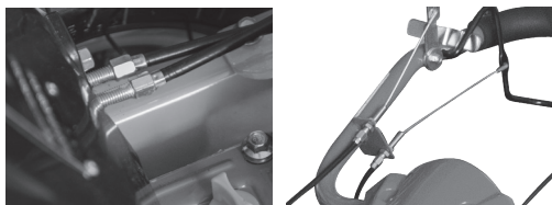
Fig. 5 – Ajuste dos cabos
