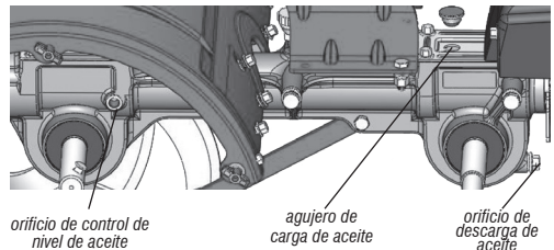
Fig. 8 – Posición para carga y descarga de aceite
