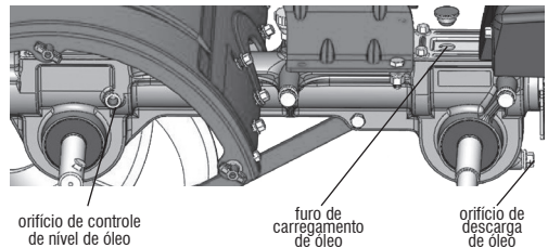
Fig. 8 – Posição para carga e descarga de óleo
