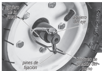
Fig. 6 – Instalación de las ruedas
