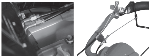
Fig. 5 – Ajuste de los cables
